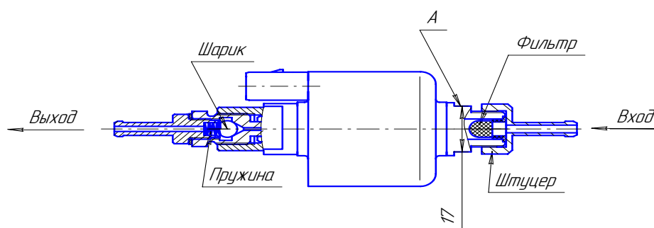
Рис.12 – Топливный насос
