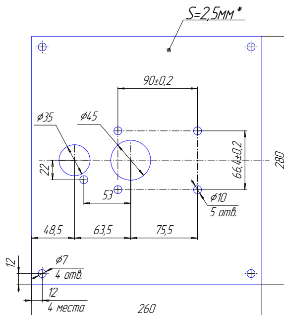
Рис 7- Пластина монтажная
