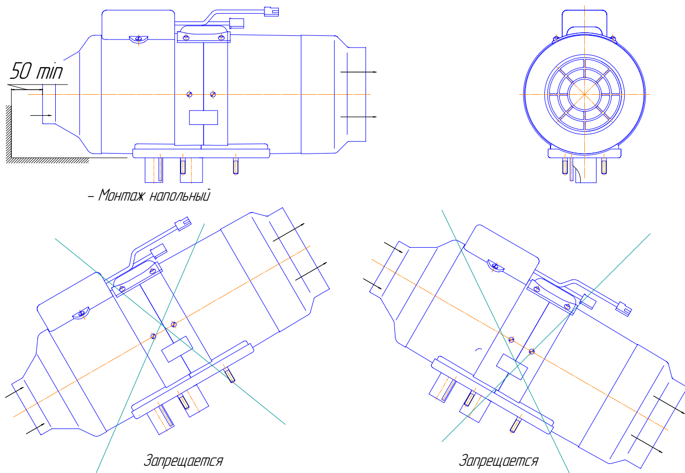
Рис. 5 – Установка нагревателя
